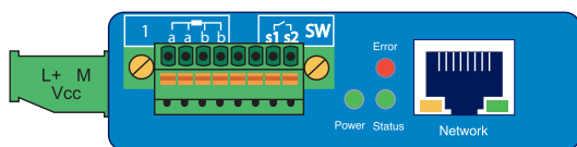
PT100 4 Draht
