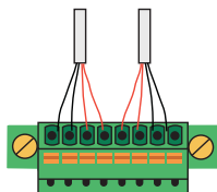
PT100 4 Draht
