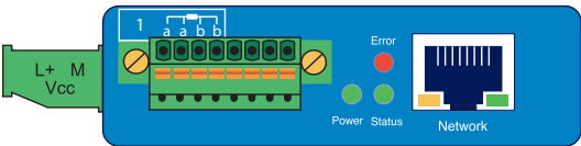
PT100 4 Draht
