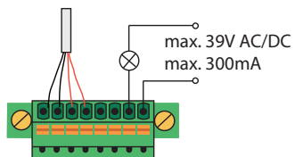
PT100 4 Draht
