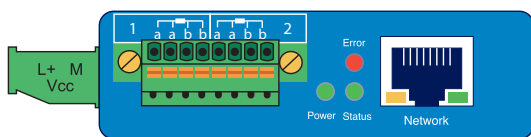
PT100 4 Draht
